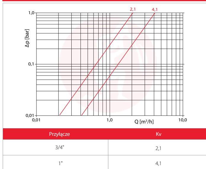
Strata ciśnienia (dla zestawu z przykładowym wodomierzem)
